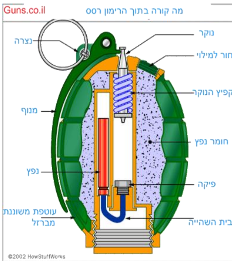
152. תרשים מבנה פנימי של רימון יד מיילס 4.
