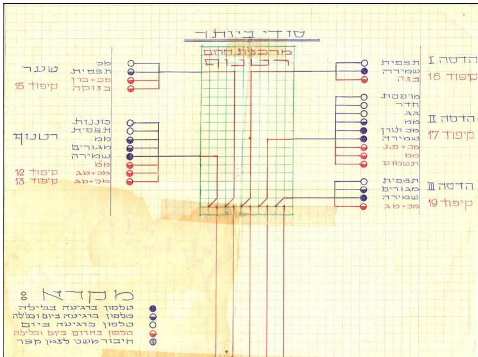
177. תרשים קשר קווי 'מקורי' קיפודי הצפון "סודי ביותר".
