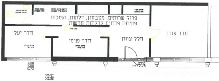
תכנית הריסה ופרוקים
