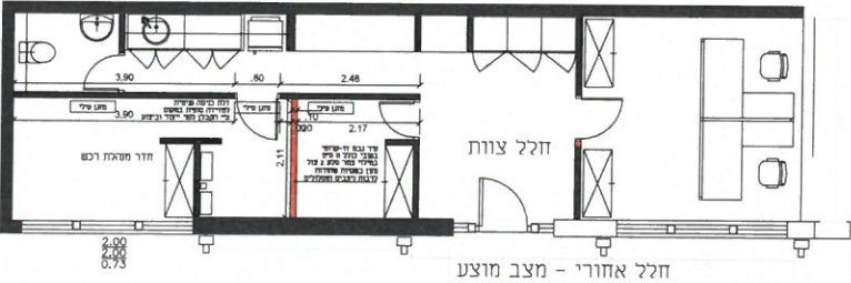
תכנית בינוי - שלב אי
